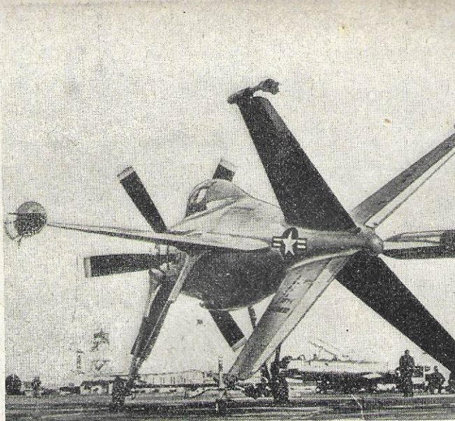
Senkrecht starten und landen kann diese neue Lockheed Jagdmaschine der US-Marine. Hier wird sie mit einem Fahrgestell zum Start geschoben, wo sie dann senkrecht auf die vier Stoßdämpfer des Leitwerks aufgestellt
