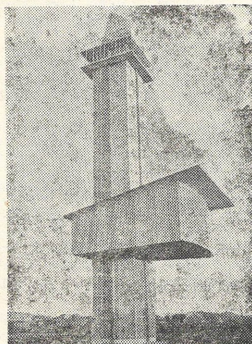
Ein 35 Meter hoher Radarturm, mit dessen Hilfe man hofft, die Schlechtwetterlandefolge von sechs Minuten auf drei Minuten verkürzen zu können, wurde kürzlich auf dem Hamburger Flughafen Fuhlsbüttel in Betrieb genommen. Das Gerät erfaßt mit Sicherheit alle Flugzeuge im Umkreis von 90 Kilometer und zeigt gleichzeitig Höhe, Geschwindigkeit und Entfernung an. (AND)
