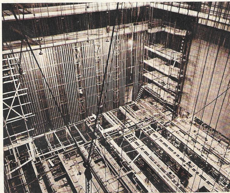
Die grandiose technische Einrichtung der Bühne zeigt dieses Bild. Der Szenenwechsel kann durch horizontale und vertikale Bewegung sowie durch eine Drehbühne bewirkt werden.
