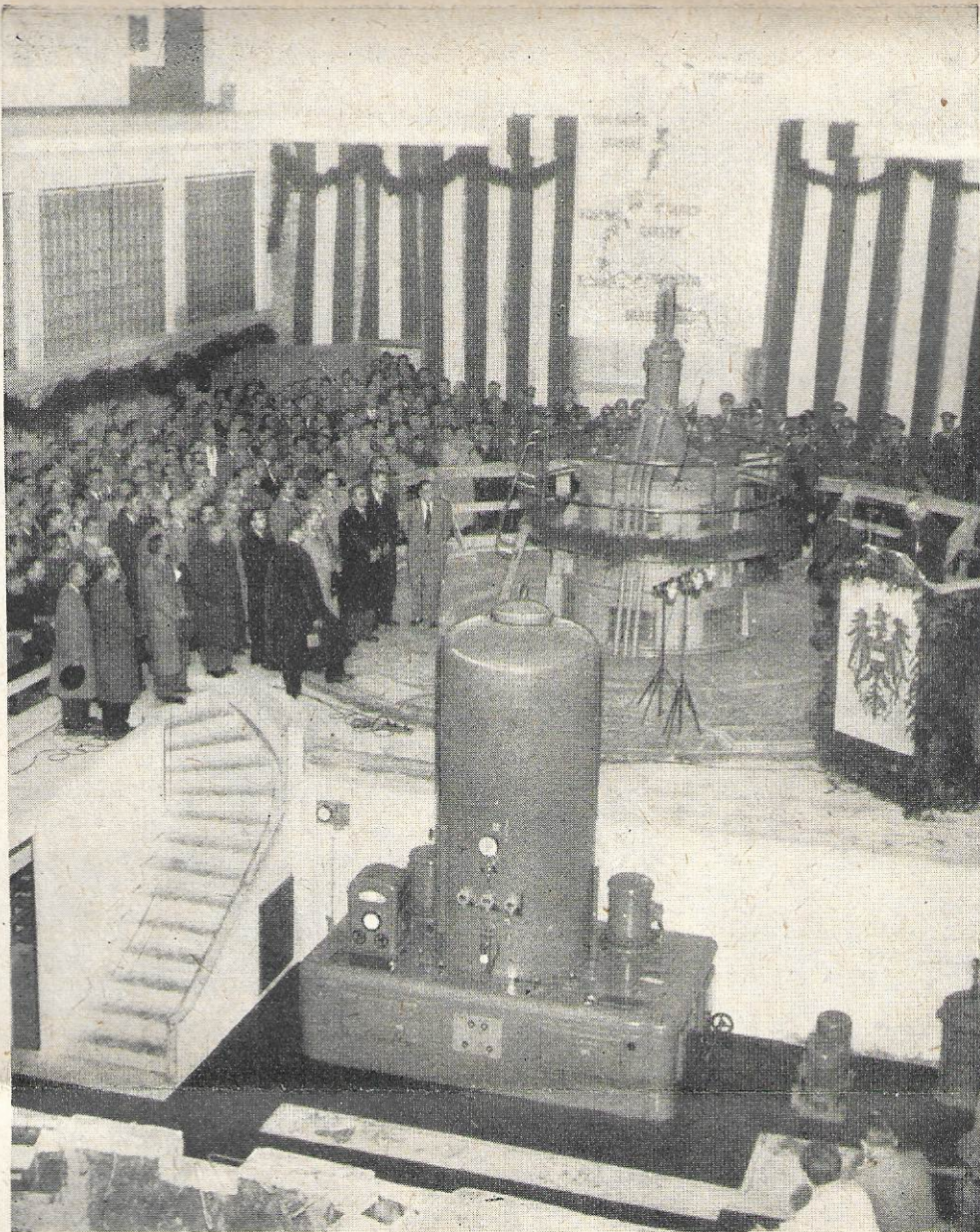
Der erste Generator des neuen Ennskraftwerkes Rosenau wurde kürzlich in Betrieb genommen. Der Feierlichkeit wohnten Bundesminister Waldbrunner sowie Vertreter der Bundesregierung und der amerikanischen Wirtschaftsmission bei, die für den Bau der fünf Ennskraftwerke namhafte Beträge zur Verfügung gestellt hat.
