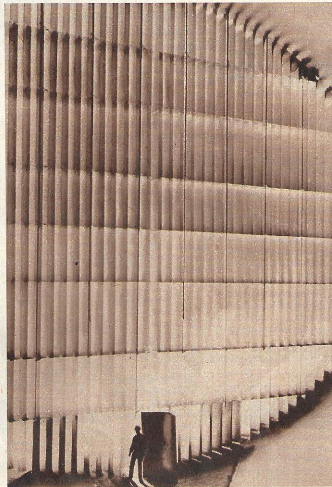
Zehnmals schneller als der Schall werden die Strömungen sein, die in dem neuen Windtunnel in Tullahoma erprobt werden sollen. Links die gigantische Schaltanlage, oben links die Ansicht des Windtunnels mit einem System von Stützkäufen, die den Luftstrom „ums Eck“ ablenken können.
