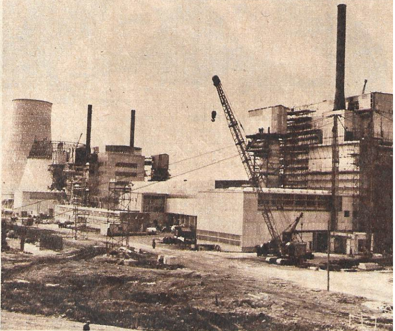
Im nächsten Jahr wird es in England bereits Atomstrom geben. Die Arbeiten an dem Atomkraftwerk in Calderhall machen gute Fortschritte. Der Thermoreaktor Nr. 1 ist fast fertiggestellt. In der Mitte erkennt man einen seiner vier Wärmeaustauscher, links einen der riesigen Kühltürme.
