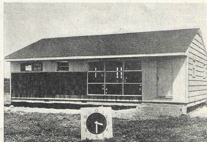
Das Aufstellen eines → Hauses aus vorfabrizierten Bauteilen in acht Stunden zeigen die nebenstehenden Bilder. Oben: Um 7 Uhr bringt ein Lastwagen die Bauelemente zur Baustelle. Mitte: Kurz nach 9 Uhr sind die Außenwände aufgestellt. Unten: Um 1/4 Uhr ist das Haus im Rohbau bereits fertig.
