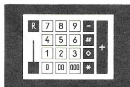
Alle Maschinen d. Modellgruppe 122 stehen auf Wunsch auch mit drei Nullentasten bereit
