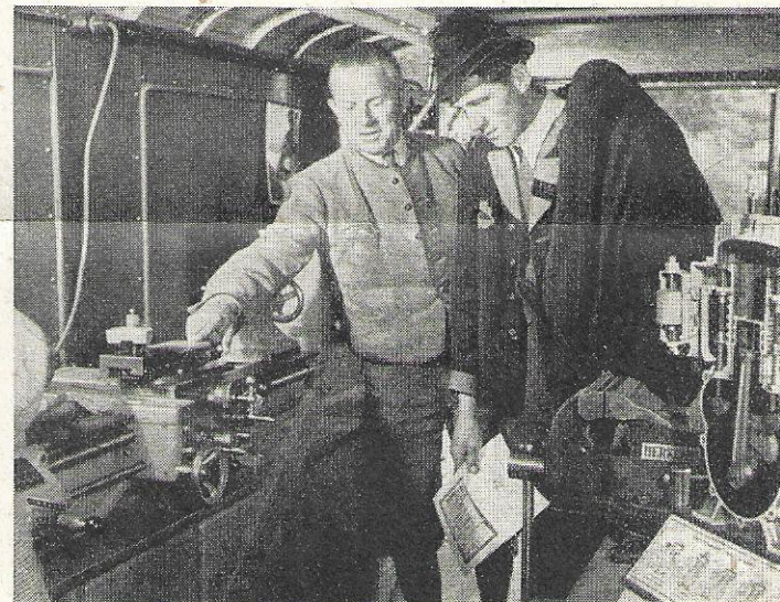
Das dreitägige Kursprogramm umfaßt theoretischen und praktischen Unterricht in Metallbearbeitungskunde, Treibstoff- und Schmiermittelkunde sowie Pflege des Motors.
