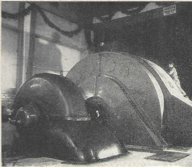
Der Generatorsatz 1 und die Turbine in der Maschinenkaverne. Die Anordnung im Bergesinnern gestattet es, das Gefälle des Wassers besser auszunützen und einen um 10% höheren Nutzeffekt zu erzielen.
