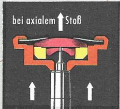
So schützt die Junghans-Stoßsicherung bei seitlichen und axialen Stößen die Zapfen und Steine der Unruh wirksam gegen Bruch.
