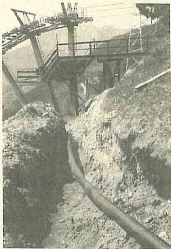
Der Kanal führt in drei Metern Tiefe.
